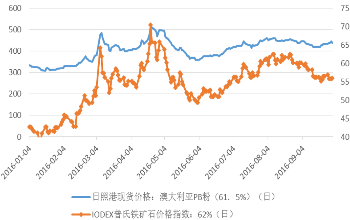
铁矿石价格
